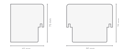
Randholz Bordure de bois Kämpfer / Pfosten Travers / Montant
