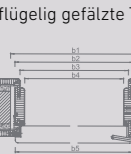
Horizontalschnitt Futter (RF)
