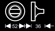
Badverriegelung EZ 1332 – BAD Farbe: Edelstahl matt
